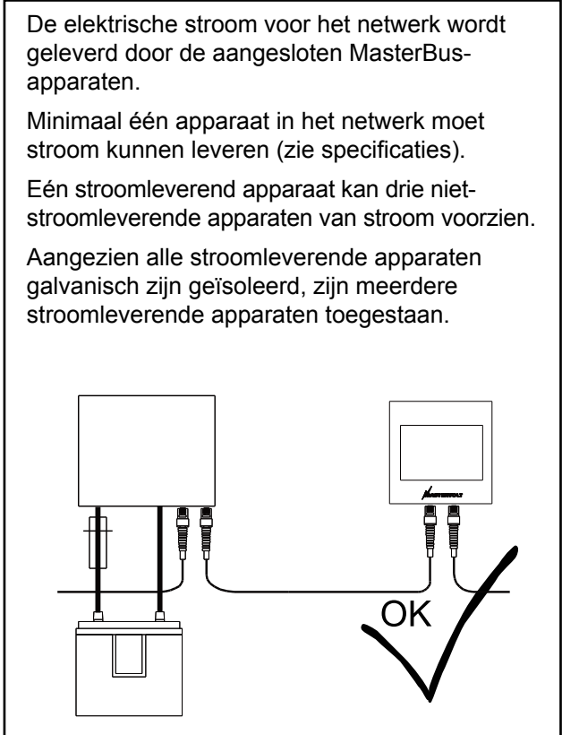
Afbeelding 6: Voeding
