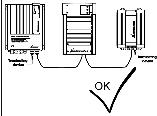
Figure 5 : Deux (2) terminateurs
