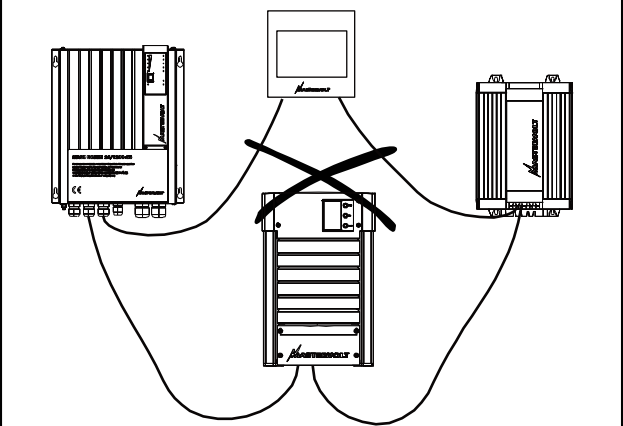
Figure 7 : Pas de réseaux en anneau
