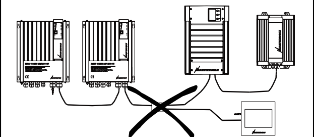
Figure 8 : Pas de couplages en T
