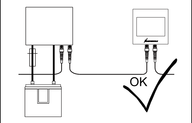
Figure 6 : Alimentation électrique
