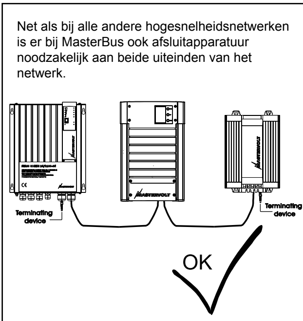
Afbeelding 5: Twee afsluiters
