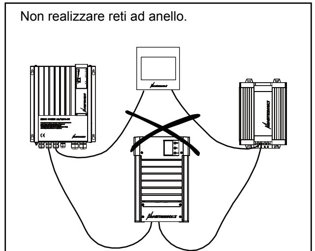
Figura 7: Reti non ad anello
