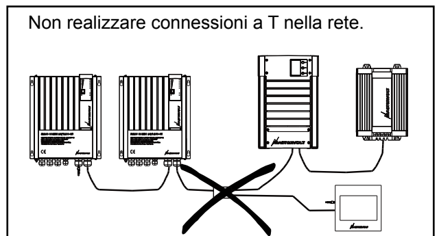
Figura 8: Connessioni non a T
